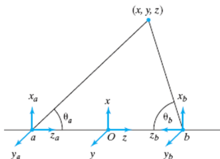
图 13.10: 同核双原子分子的坐标系。
